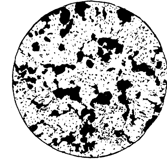
ТА 8 пта и троостита х500
